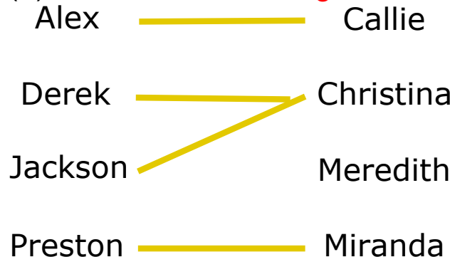
(d) Not a matching
