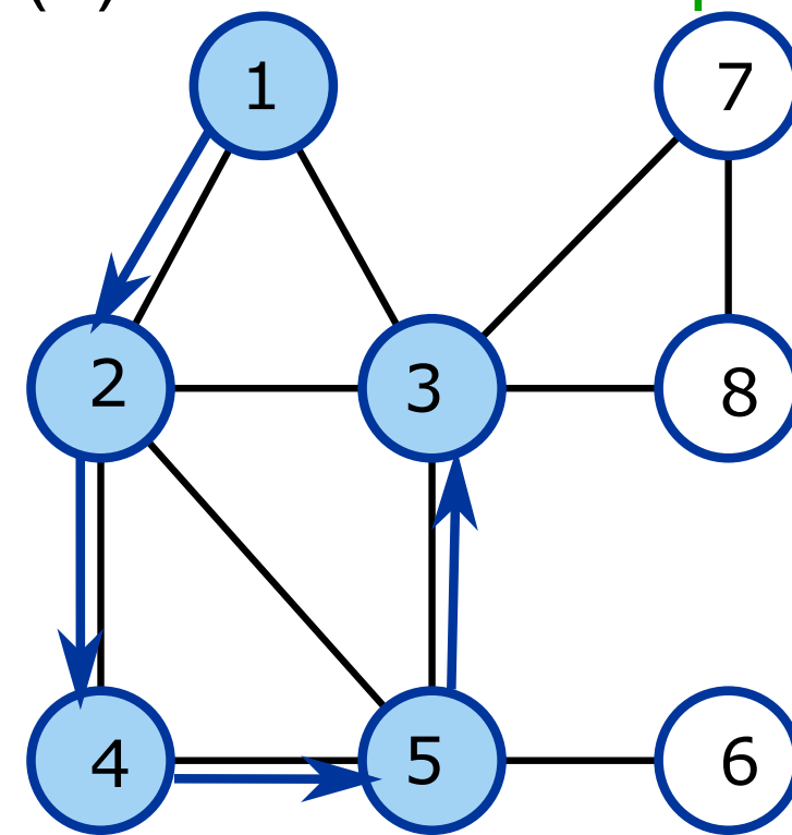
(d) Simple path
