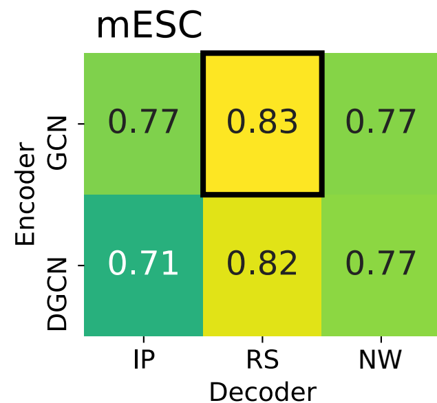
(a) 10-fold edge CV
