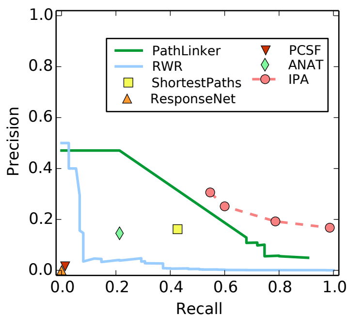
PPI Evaluation
