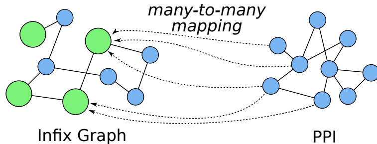
PPI Evaluation
