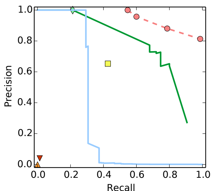
PPI Evaluation
