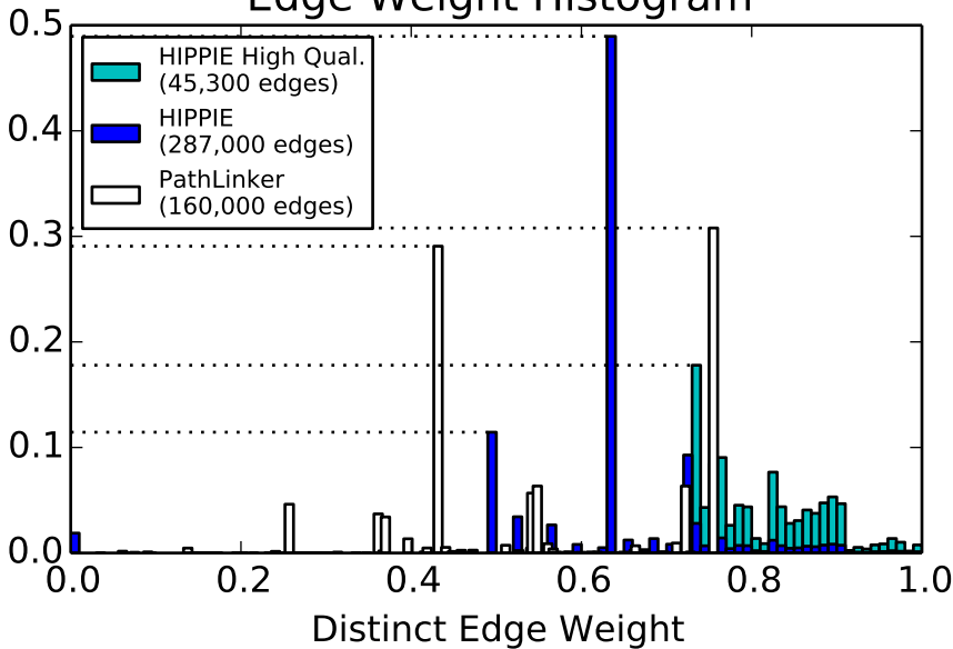
Edge Weight Histogram
