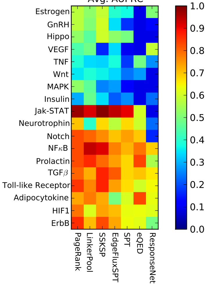
Avg. AUPRC
