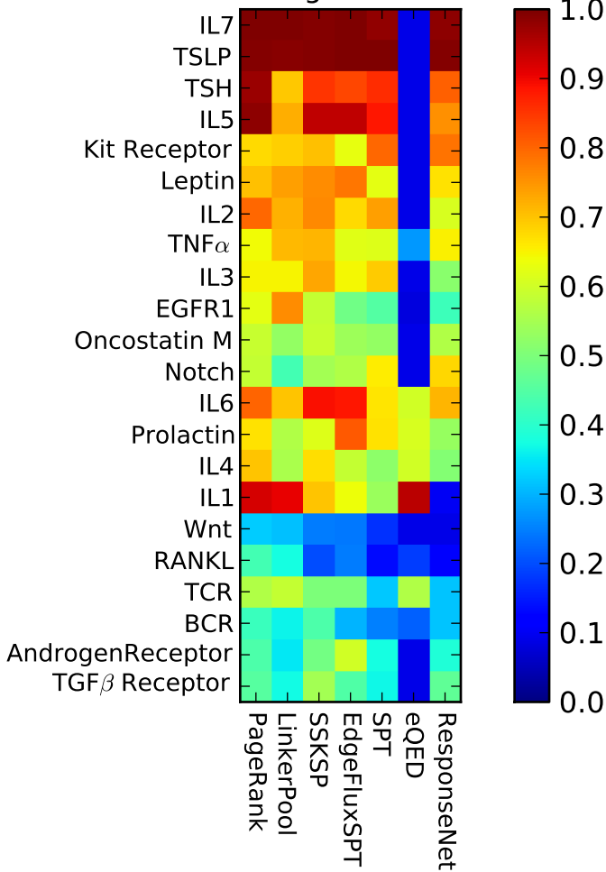
Avg. AUPRC
