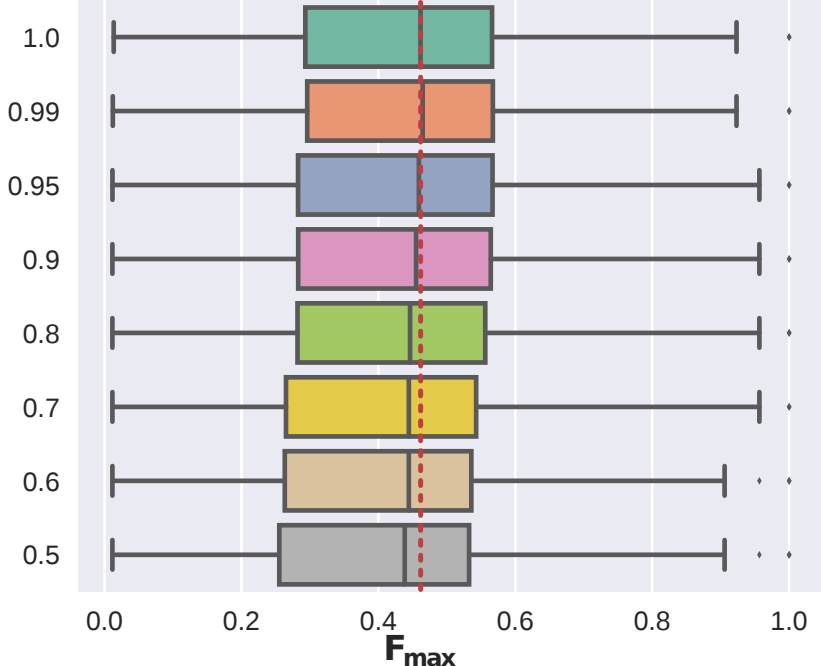
Parameter \alpha
